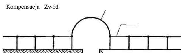
Rys. 12 Wykonanie kompensacji zwodu
