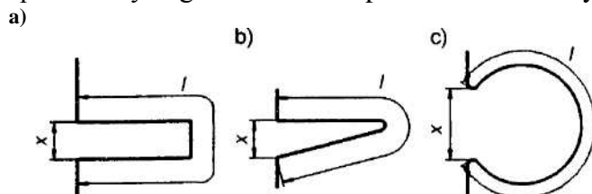
Rys. 13 Zasady pętli cofniętej ( I < 10 * x )
