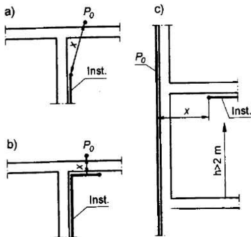
Rys. 16. Przykład zblizeń a) i b) przekrój poziomy fragmentu obiektu; c) przekrój pionowy fragmentu obiektu;
